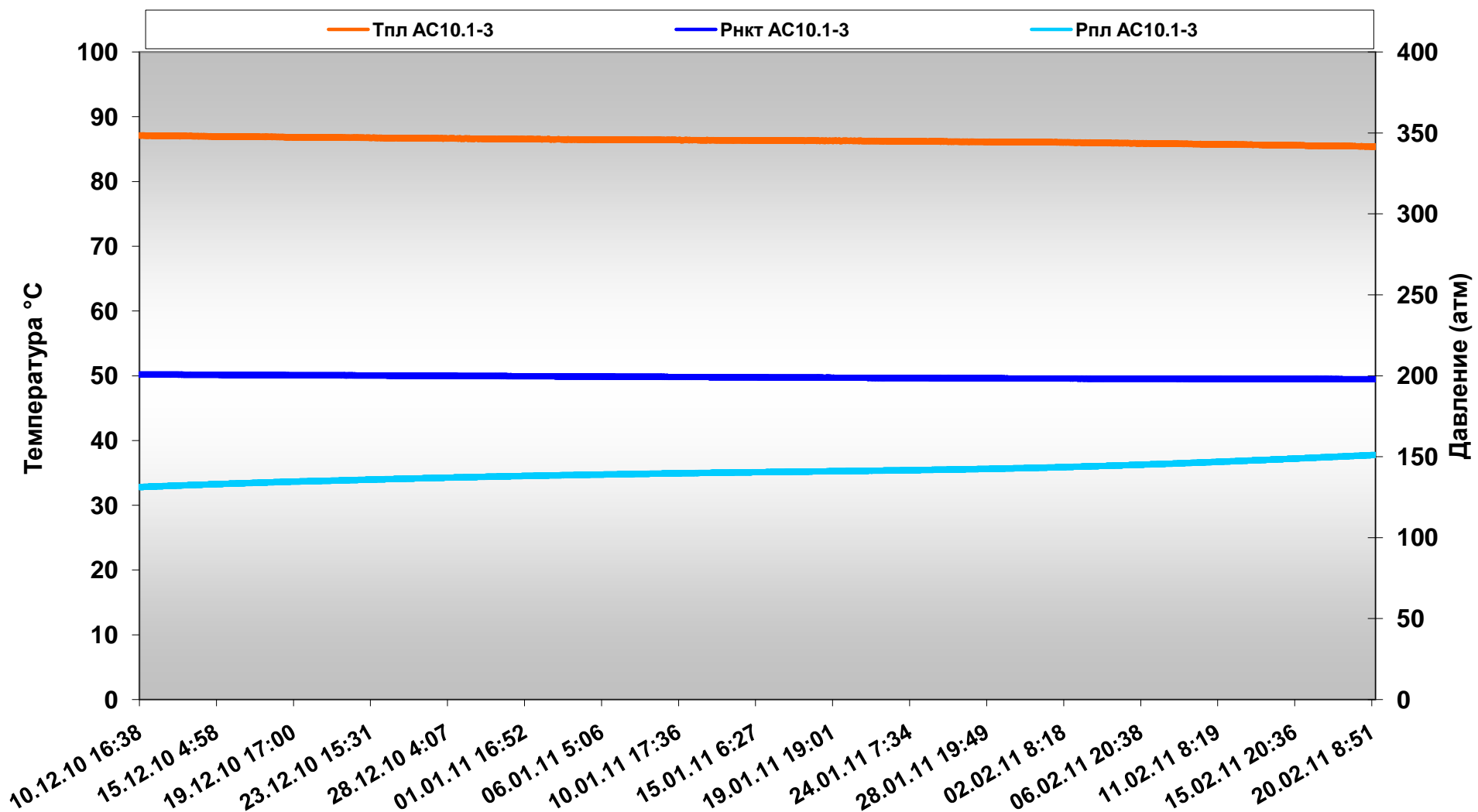
Данные с глубинного комплекса ИСДК-2G с замером давлений в режиме "on-Line" с 10.12.2010г. по 20.02.2011г. (в пьезометрической скважине между пространством в НКТ и интервалом перфорации нет сообщения)
