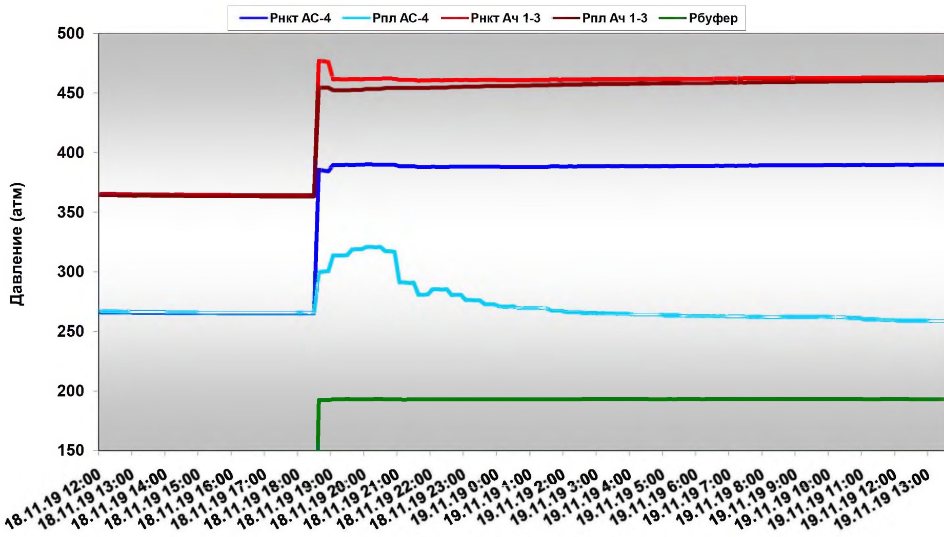
Двухпакерная компоновка с глубинным комплексом ИСДК-2G с замером давлений в режиме "on-Line" с 12ч00м 18.11.19г. по 13ч00м 19.11.19г.
