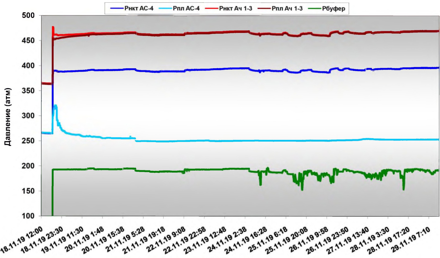
Двухпакерная компоновка с глубинным комплексом ИСДК-2G с замером давлений в режиме "on-Line" с 12ч00м 18.11.19г. по 13ч00м 29.11.19г.
