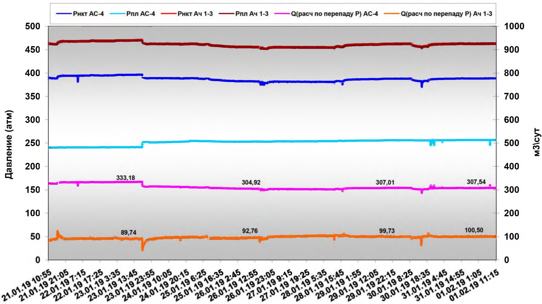
Двухпакерная компоновка с глубинным комплексом ИСДК-2G с замером давлений в режиме "on-Line" с 10ч55м 21.01.19г. по 11ч15м 01.02.19г.
