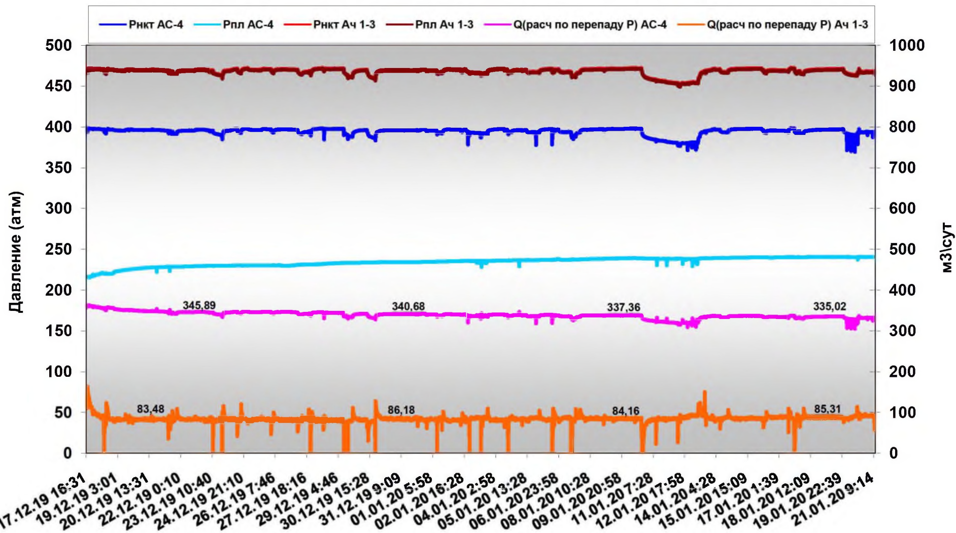
Двухпакерная компоновка с глубинным комплексом ИСДК-2G с замером давлений в режиме "on-Line" с 16ч31м 17.12.19г. по 10ч34м 21.01.20г.
