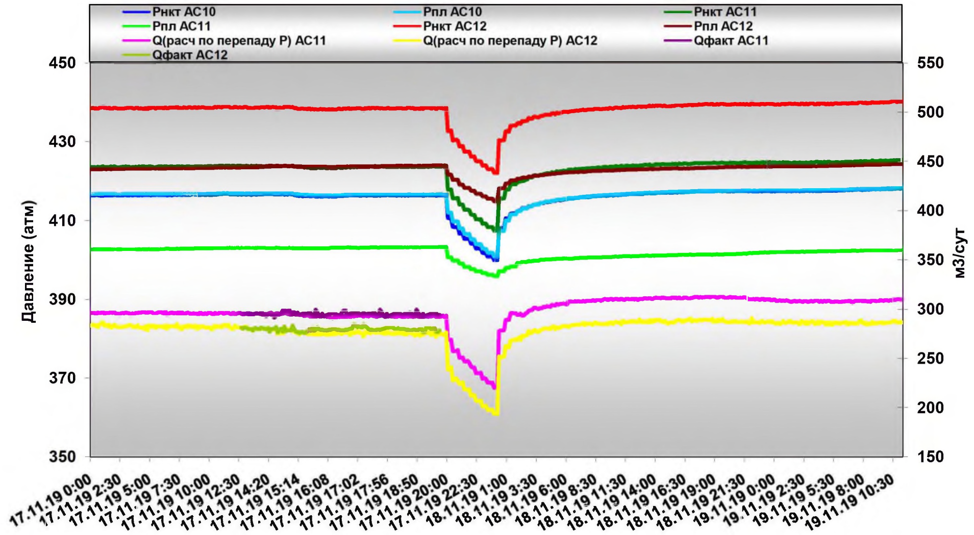
Трехпакерная компоновка с глубинным комплексом ИСДК-2G с замером давлений в режиме "on-Line" с 0ч00м 17.11.19г. по 11ч00м 19.11.19г.
